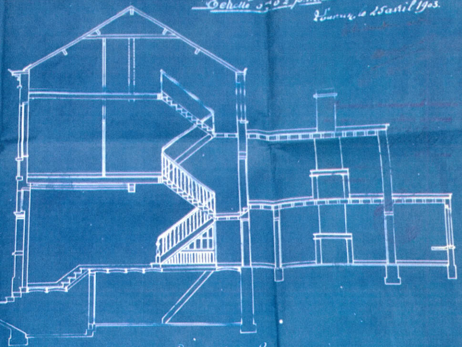
Coupe verticale
