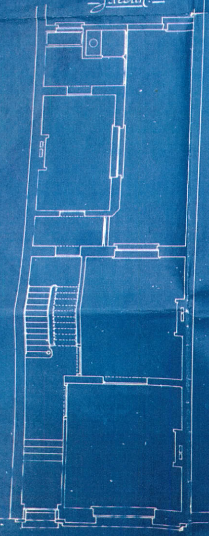
Plan du Rez de chaussée
